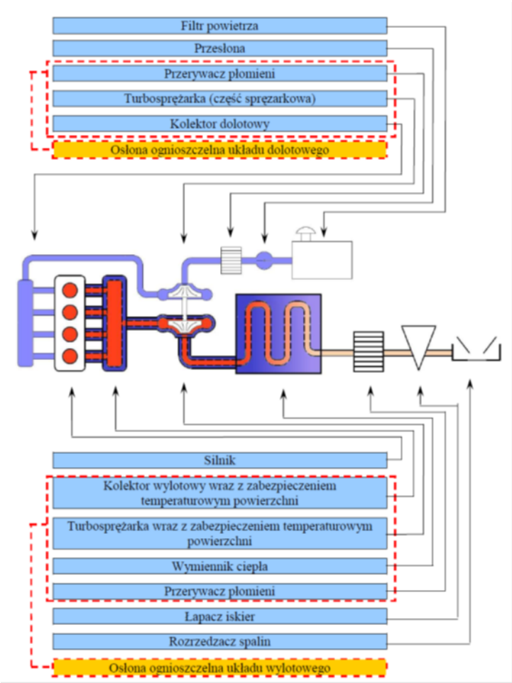
Schemat silnika spalinowego z ognioszczelnym zespołem dolotowo-wylotowym.
